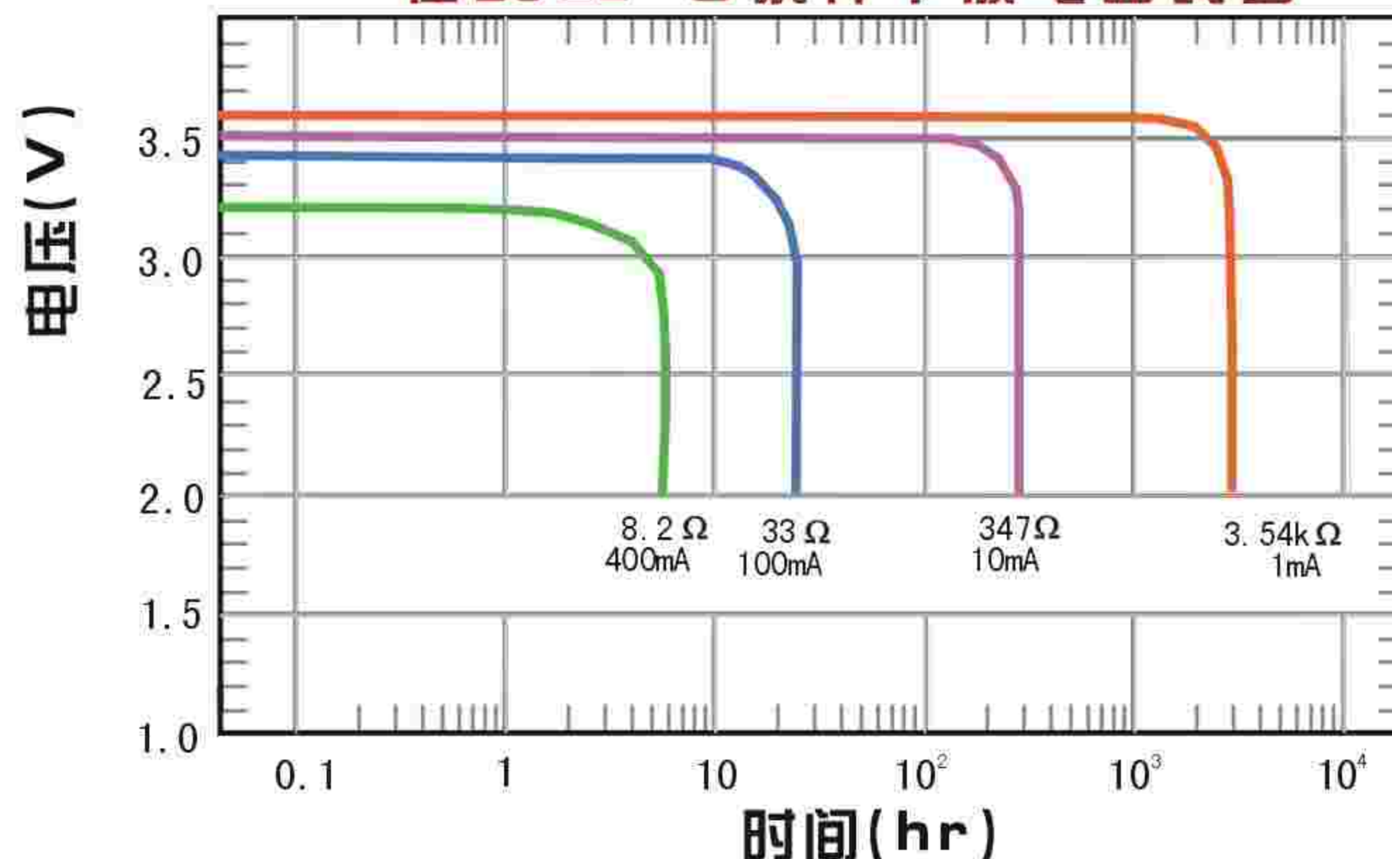
在 23 \pm 2^{\circ}\text{C} 条件下放电曲线图
